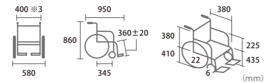
細ハイポリマータイヤ 22"×1 ブラハンドリム
