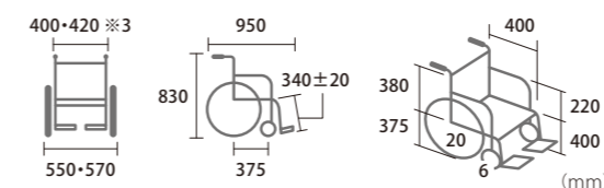
ライトタイヤ 20"×1 ブラハンドリム
