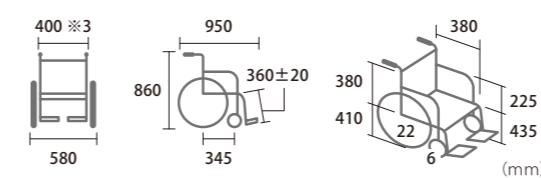
ライトタイヤ 22"×1 アルミハンドリム
