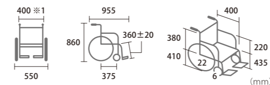
ライトタイヤ 22"×1 ブラハンドリム
